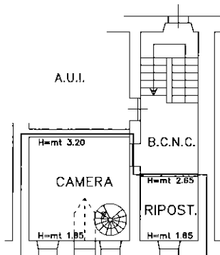
PIANO TERZO
