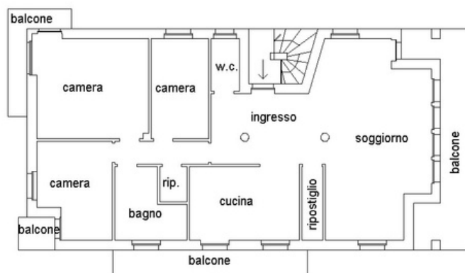
primo piano - h. m. 2.70
