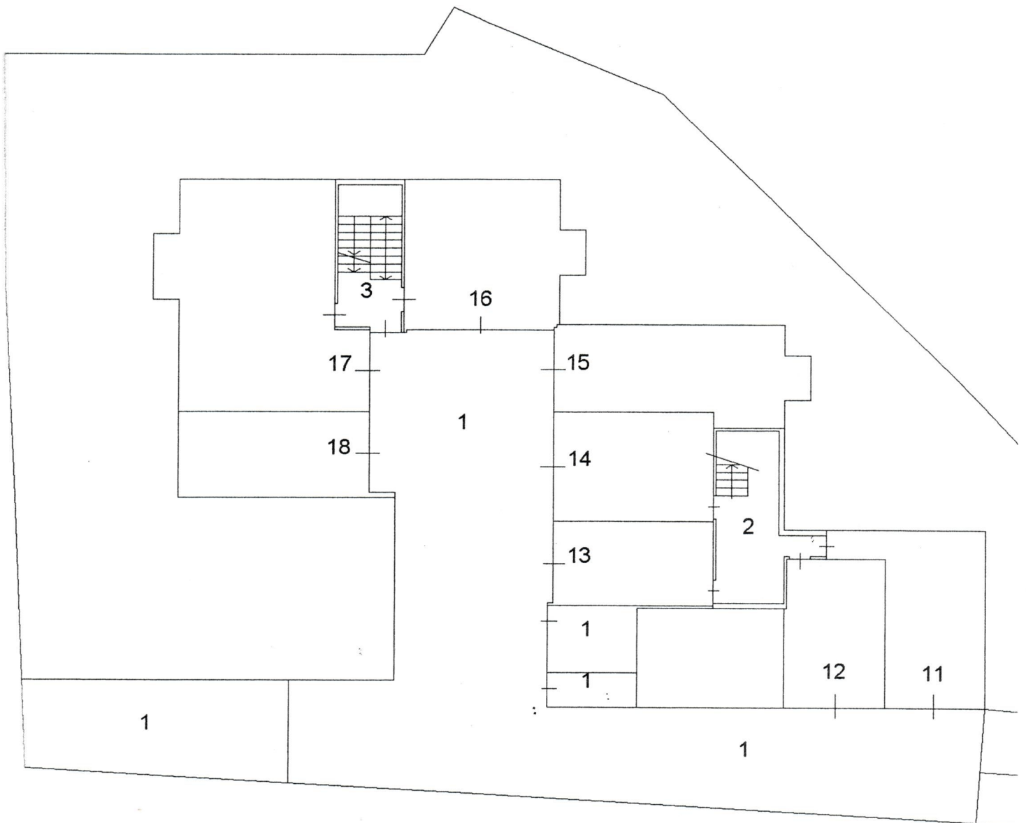
PIANO PRIMO SOTTOSTRADA
