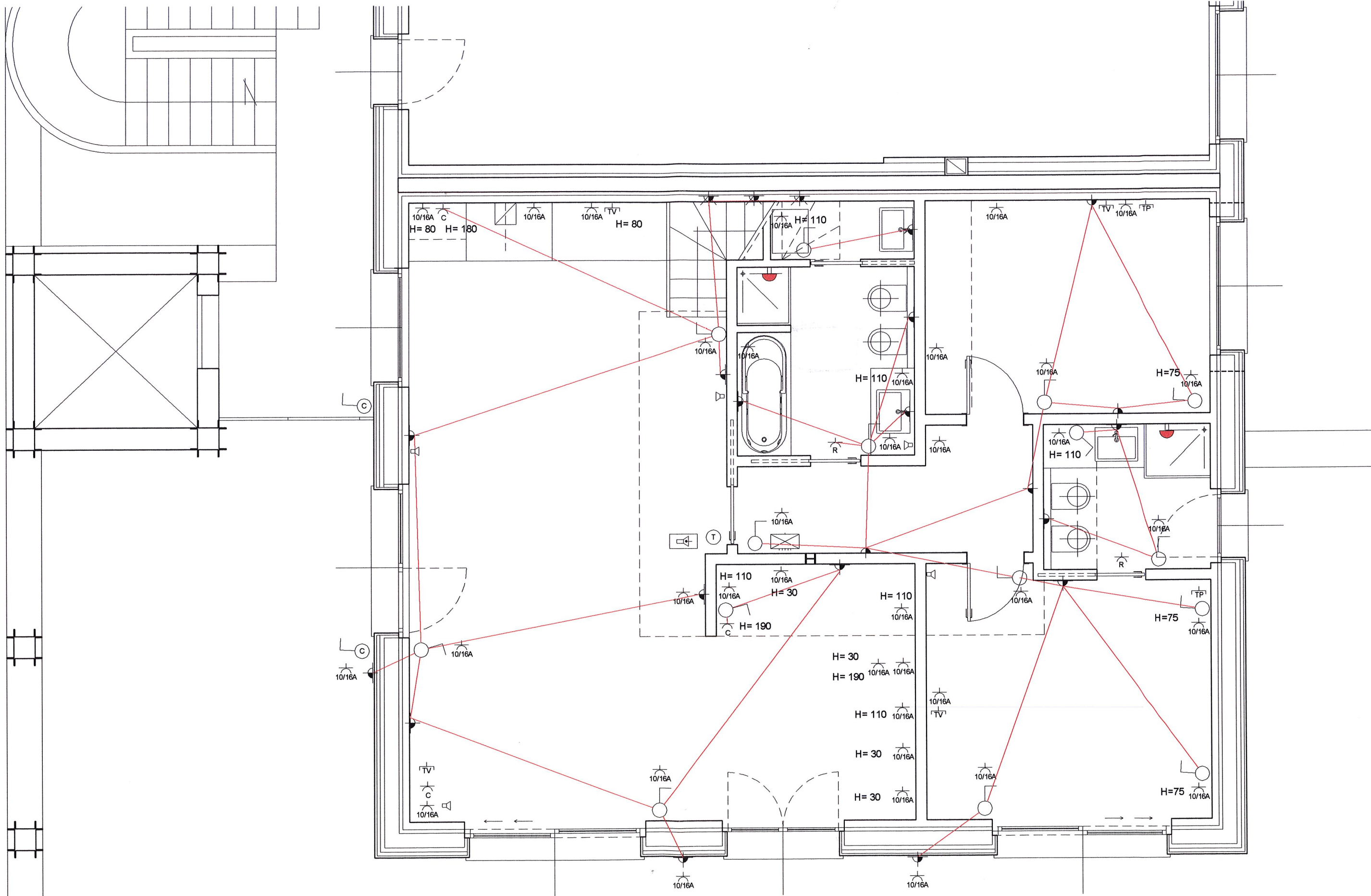
SECONDO PIANO scala 1:50
