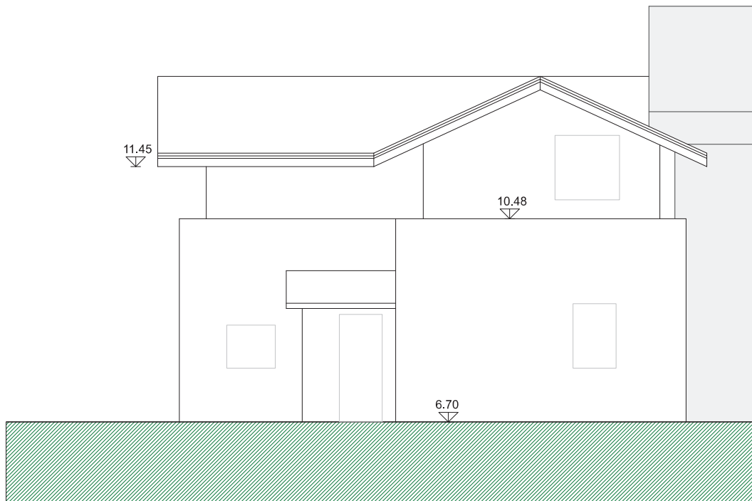
PROSPETTO SUD
