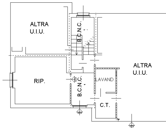
PIANTA PIANO TERRA H. 2,65m
