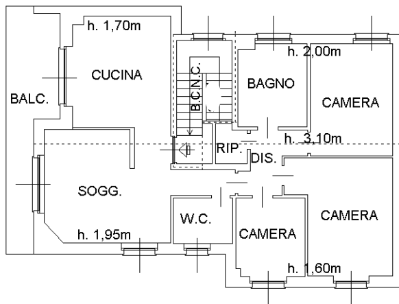
PIANTA PIANO SECONDO (Sottotetto)
