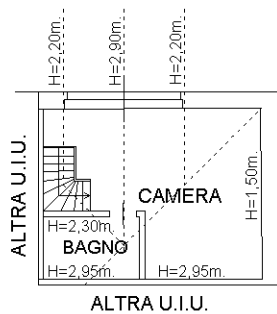
PIANTA PIANO QUARTO
