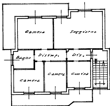
PIANO PRIMO H=mt.2,80
