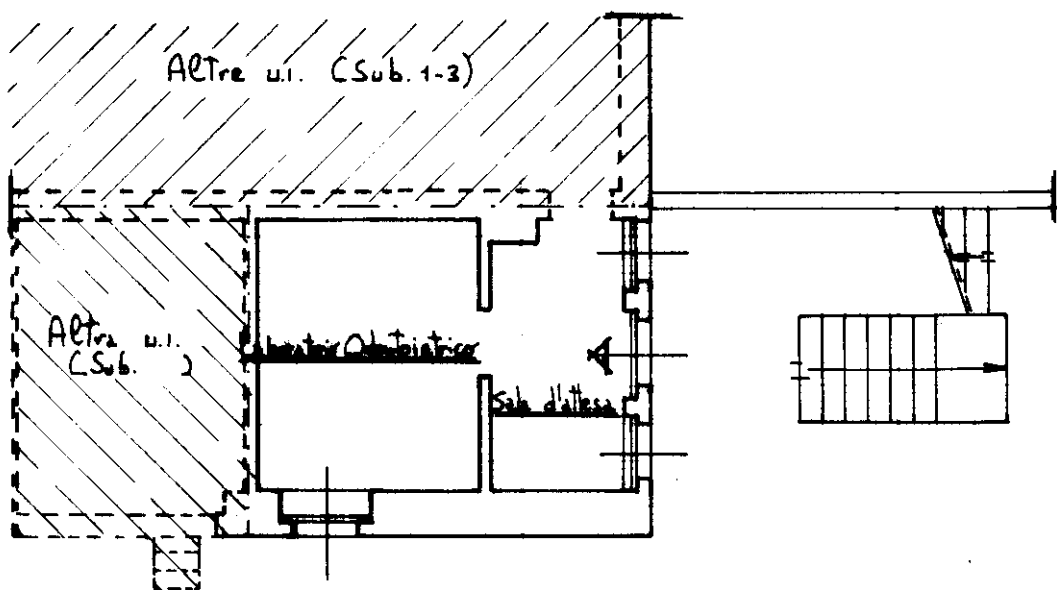
PIANTA PIANO TERRA h. = 2.75 ml
