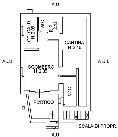
PIANTA PIANO PRIMO SOTTOSTRADA
