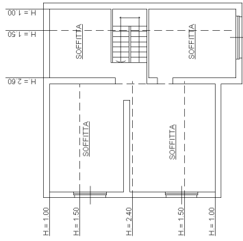
PIANO SECONDO (Sottotetto)
