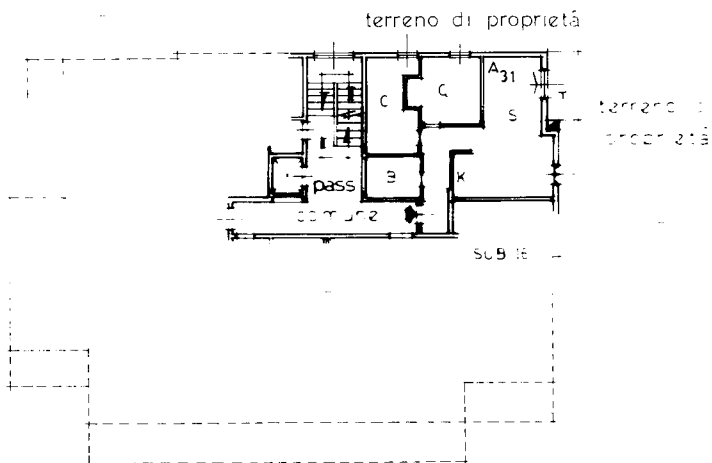
PIANTA TERZO PIANO H=m 2,50
