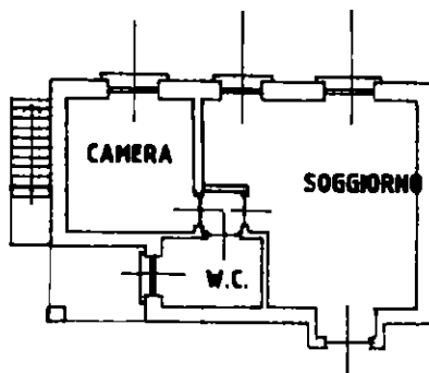
PIANO TERRENO h. 2.70
