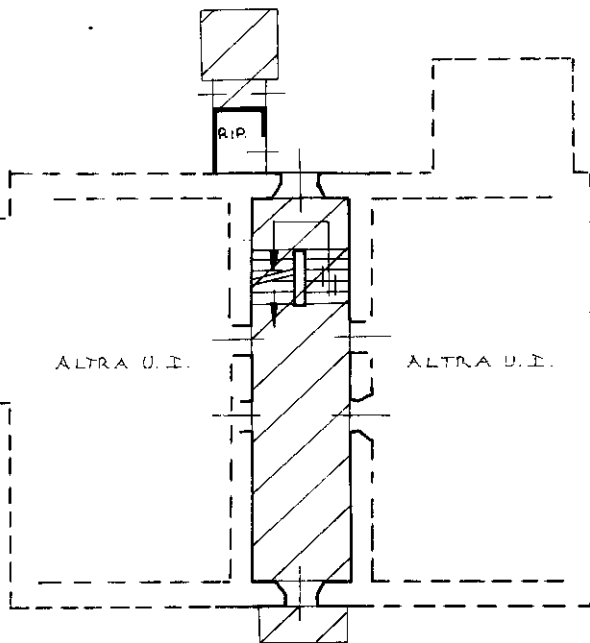
PIANO PRIMO H=220
