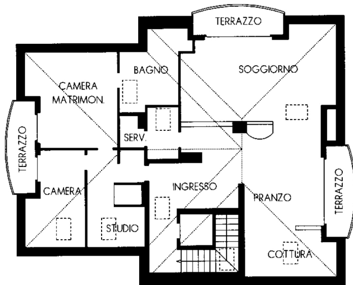
PIANO TERZO - H. 2.10/4.10
