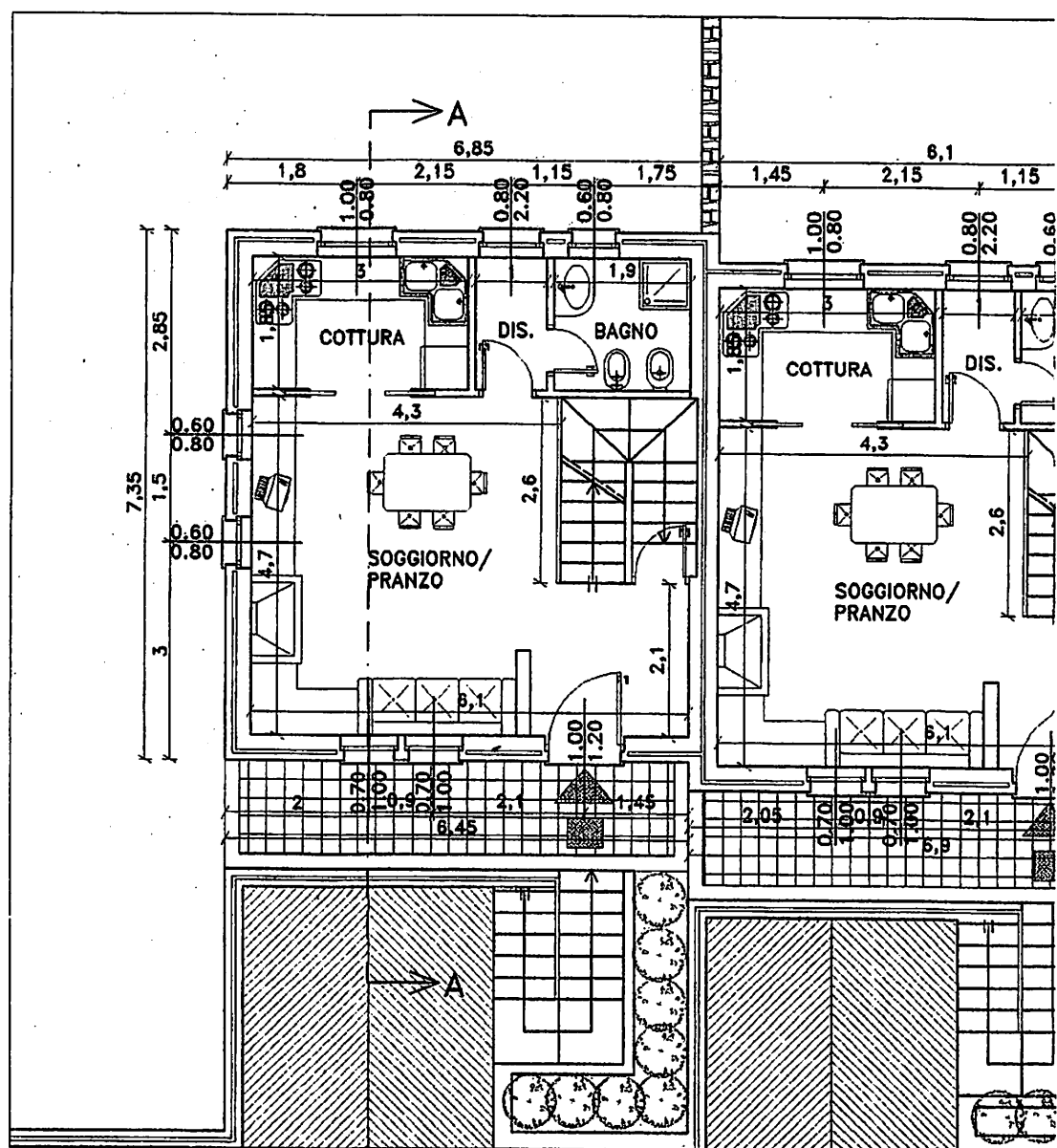
PIANTA PIANO TE
