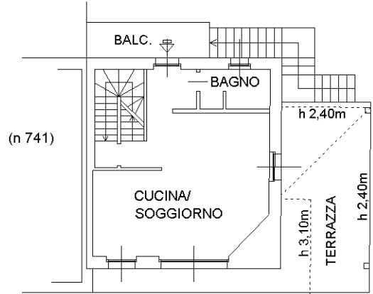
PIANTA PIANO PRIMO H. 2,70m
