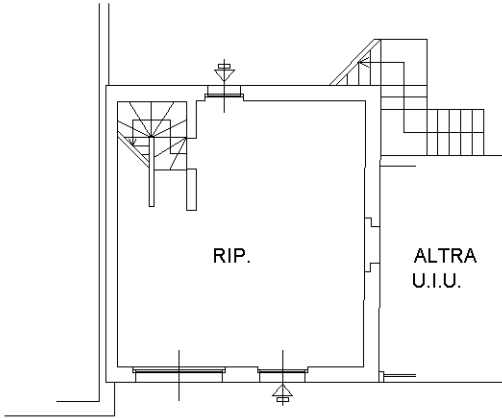
PIANTA PIANO TERRA H. 2,50m
