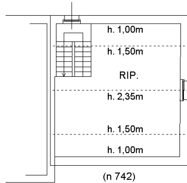
PIANTA PIANO TERZO (SOTTOTETTO)
