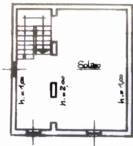
H Piano Secondo (Sottotetto)
